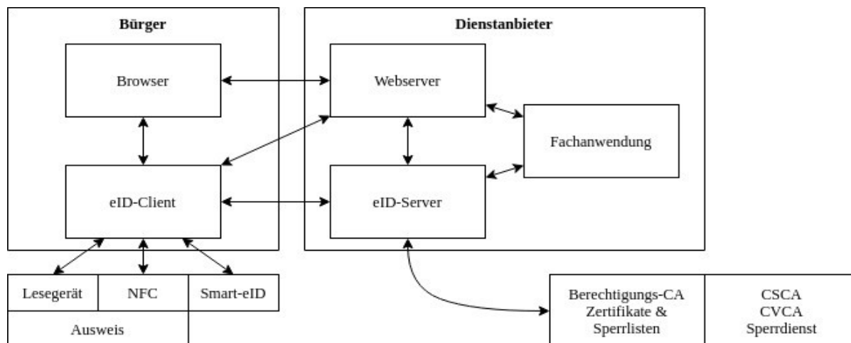
Abbildung 2: Kommunikationsbeziehungen elektronischer Identitätsnachweis
