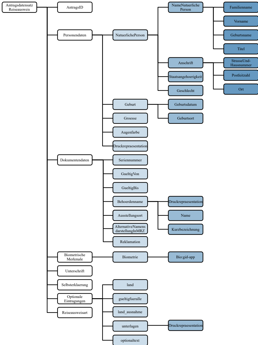
Abbildung 7: Antragsdatensatz elektronischer Reiseausweis
